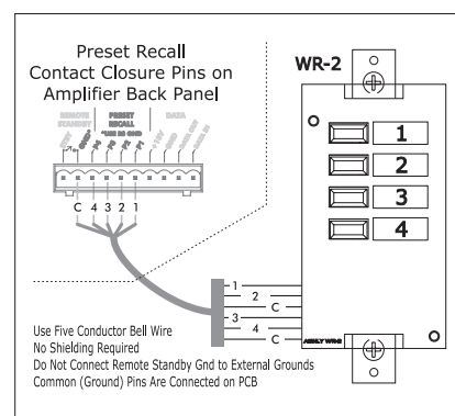
4.3 - WR-2 Wiring
