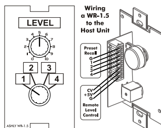
4.2 - WR-1.5 Wiring
